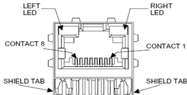
<그림 2> Ethernet 커넥터 사진 및 LED 동작 상태
