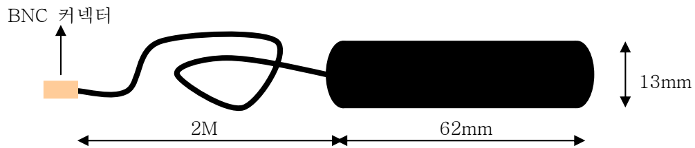
<그림 7> 원형 안테나 치수
