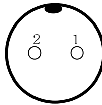
<그림 4> 전원 커넥터 핀 배치
